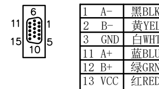
编码器接线图:
