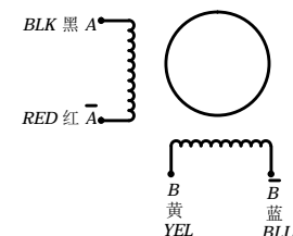
电机接线图:
